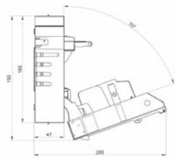
NH00 3P3P Dimensions
